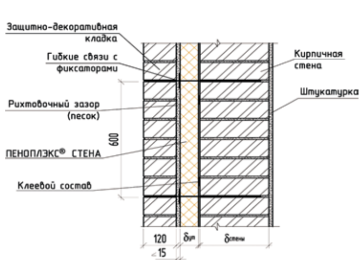
Рис. 3. Конструкция наружной стены здания № 3 (кирпич – ПЕНОПЛЭКС Стена – защитно-декоративная кладка).
