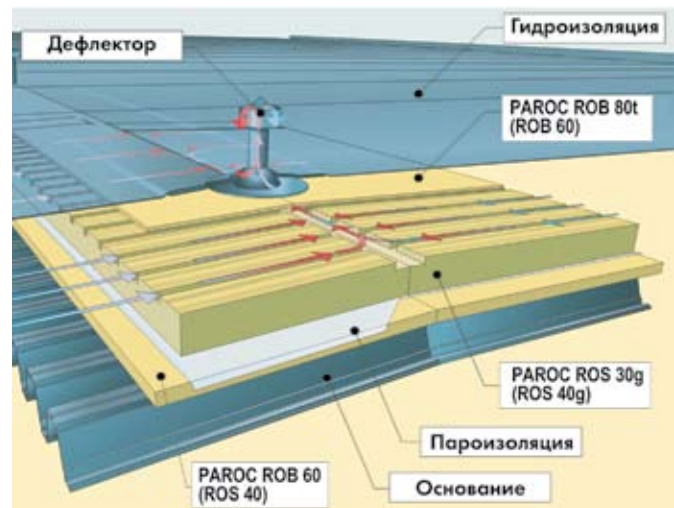
Рис. 4. Устройство системы PAROC Air
